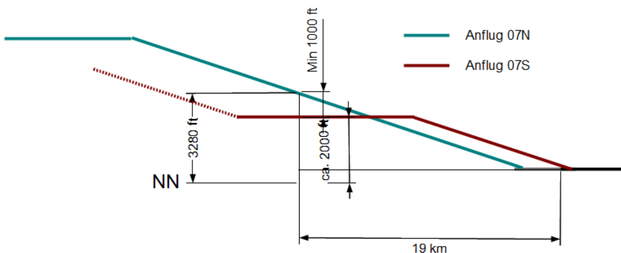
Abbildung 1: Höhenstaffelung beim Anflug bei BR07
