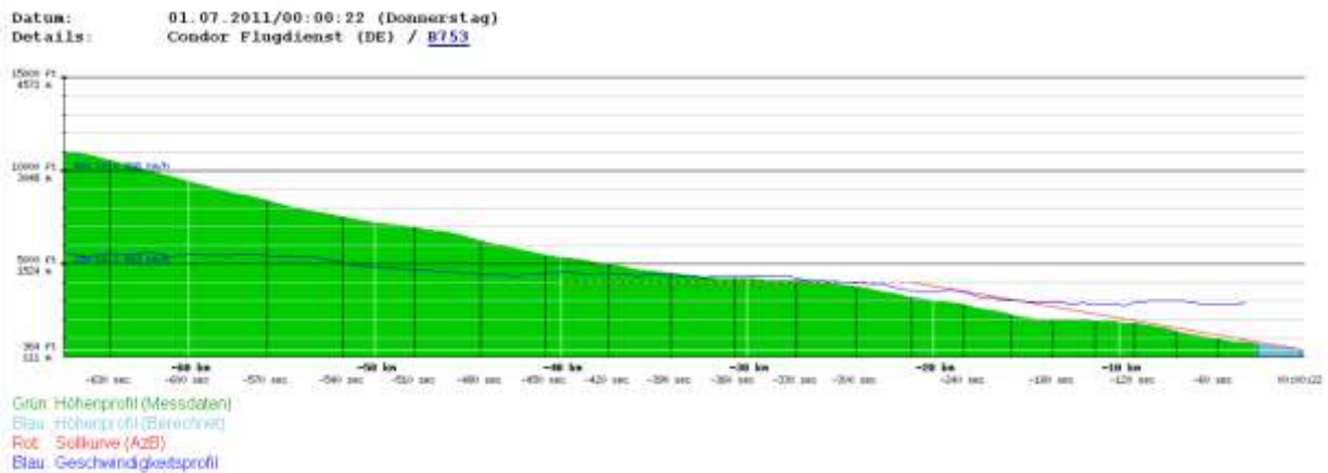
Abbildung 4: Anflug über Segmented Approach Verfahren; Quelle: DFLD
